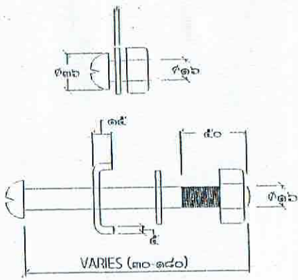
สลักเกลียว และแป้นเกลียว
